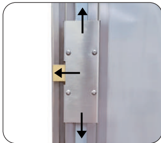
Serrure à 3 points de fermeture (de série)
