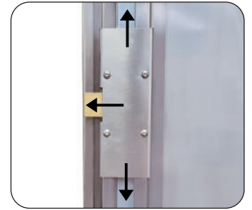
Serrure à 3 points de fermeture (de série)
