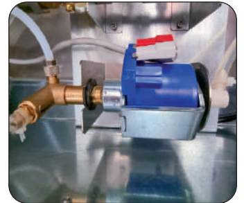
Elettromagnetico pump (standard)
