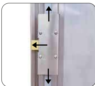
Serratura a 3 punti di chiusura (di serie)
