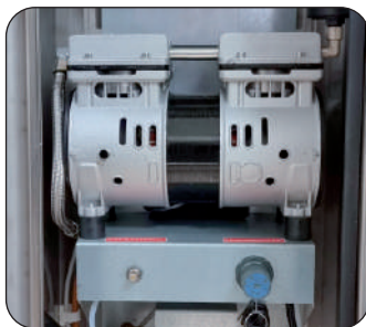
Compressore interno (di serie)
