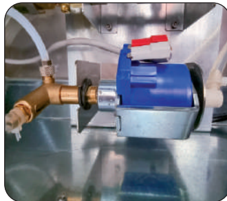
Pompa elettromagnetica (di serie)
