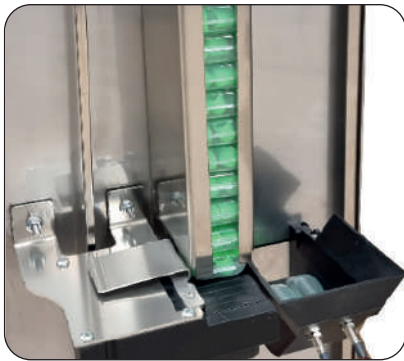
Erogatore blister tappi valvole (optional)
